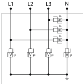
V : Varistor de alta energía t* : Sistema de desconexión térmica
