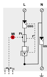
DACN1-25CVGS-11
