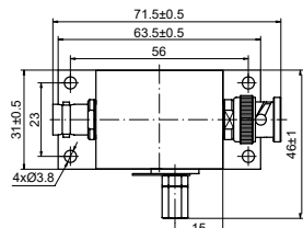
CXP-B/MF
