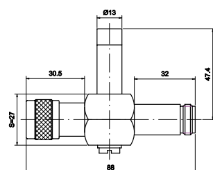
PRC1800-N/MF
