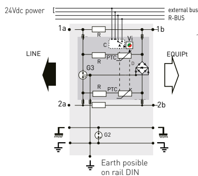
DLATS1-xxx DLATS1-xxx/R Line continuity if plugout
