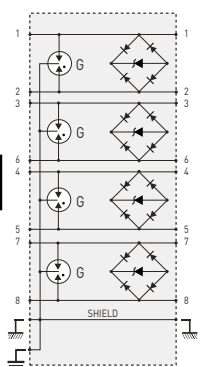
MJ8-POE-A
