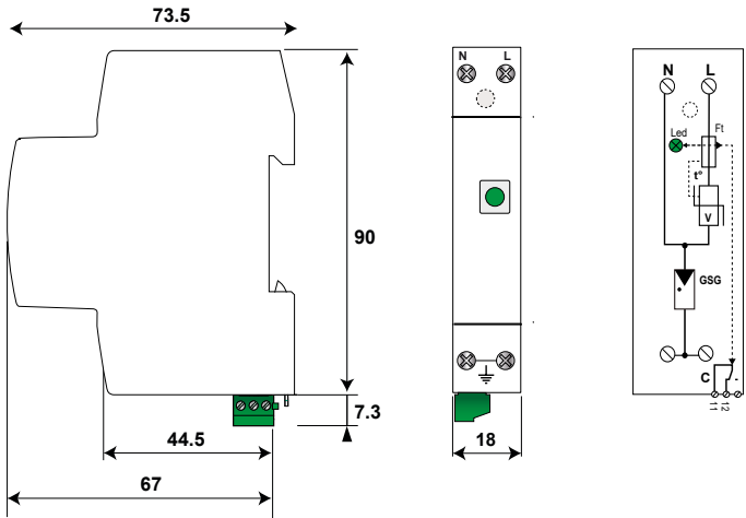
DACN15S-P11-xxx
